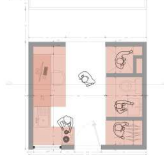
Planta vivienda individual de 12m 2 Esc. 1/25
