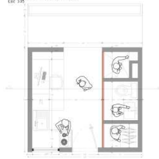
Planta vivienda individual de 12m 2 Esc. 1/25
