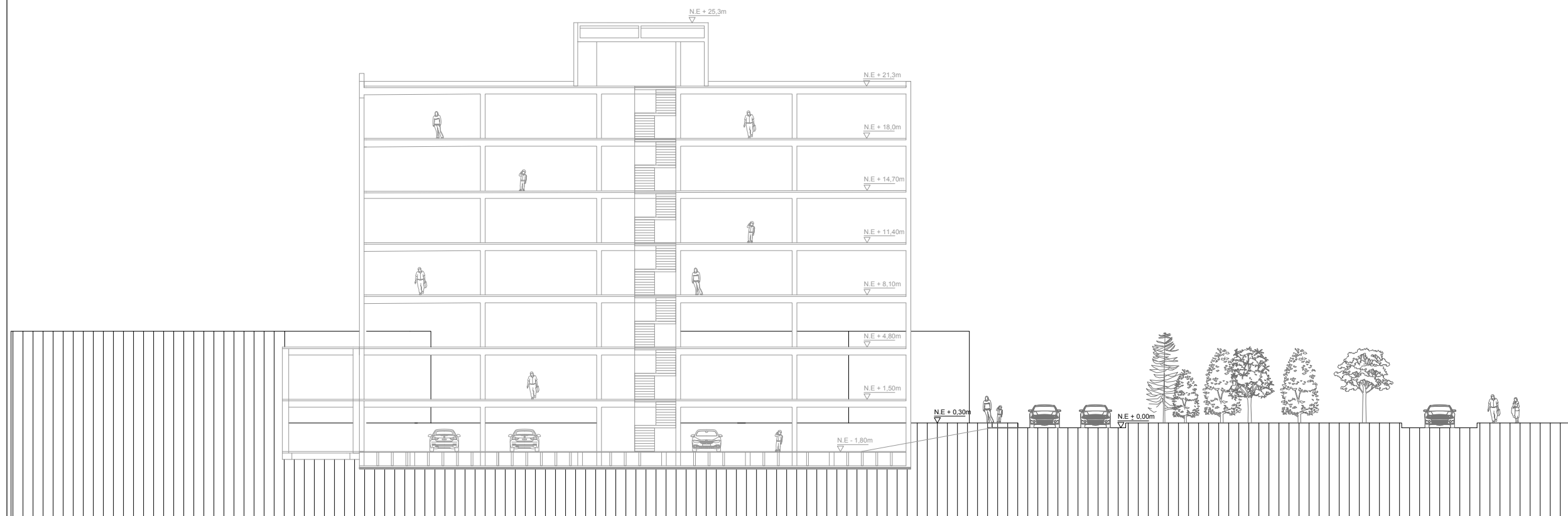
CORTE A-A'
